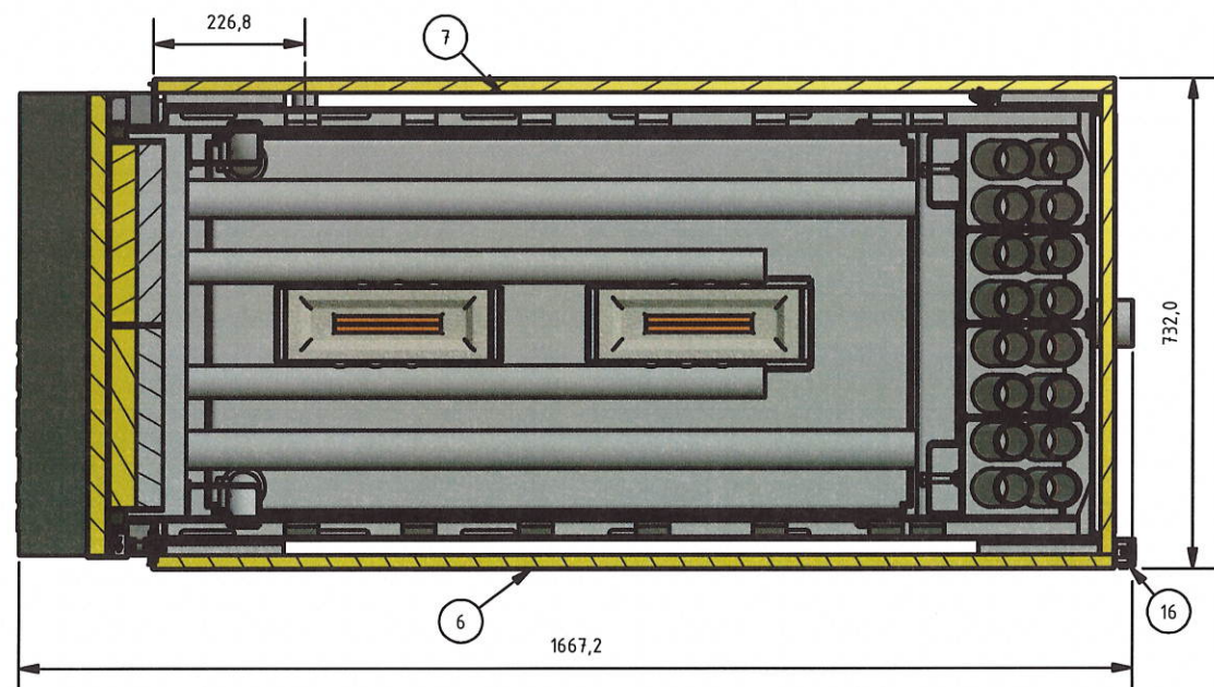
B-B ( 1 : 12 )
